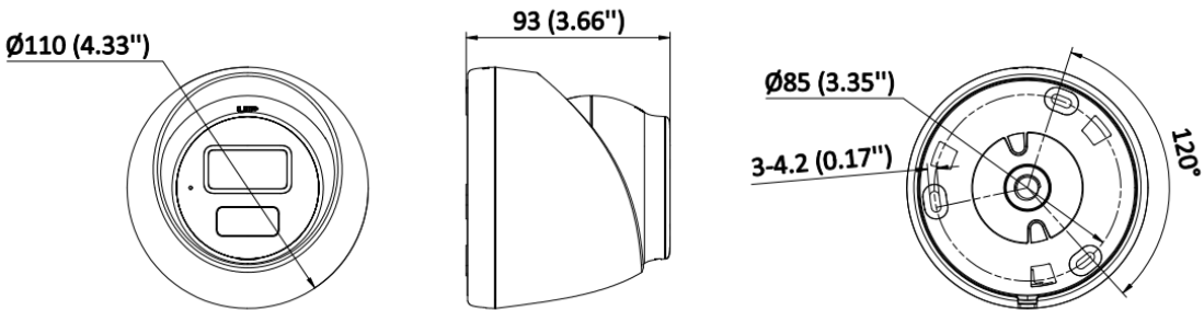
Unit:mm (inch)
