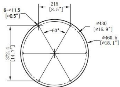
推荐打孔安装尺寸图
