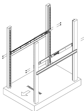
② Installare i binari esterni
