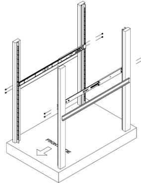
② Pasang Rel Luar
