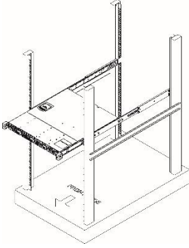
③ تثبيت الخادم على الحامل
