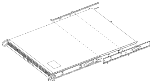
① Szerelje fel a belső síneket a szerverre
