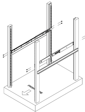
② Installer les rails extérieurs
