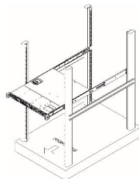
③ Installeer de server in het rack
