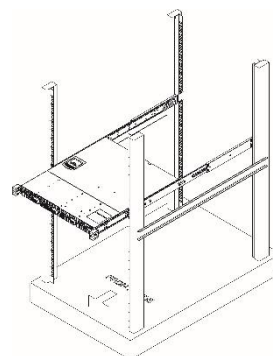
③ Installare il server nel rack
