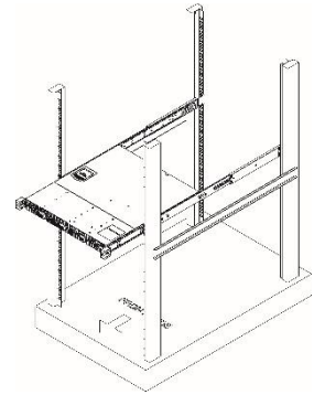
③ Sunucuyu Rafa Kurun
