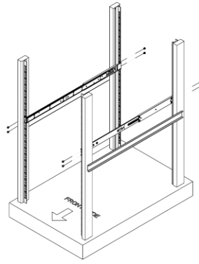
② Встановіть зовнішні напрямні
