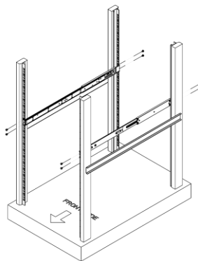
② Instalați șinele exterioare
