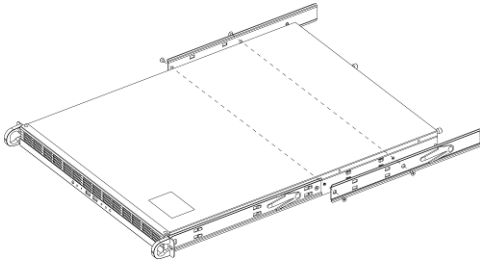
① Sunucu ve İç Rayları Sabitleyin
