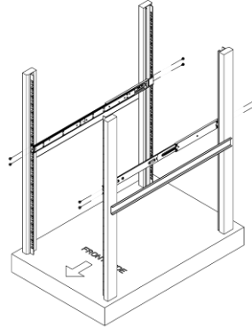
② Dış Rayları Takın
