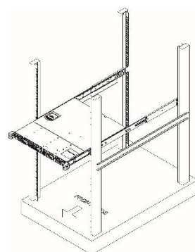
③ Instalați serverul în raft
