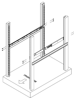
② Szerelje fel a külső síneket
