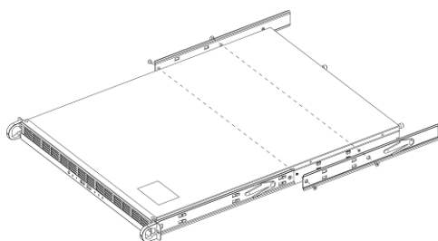
① Fixați serverul și șinele interioare
