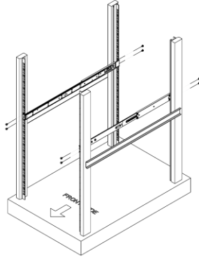
② تثبيت القضبان الخارجية
