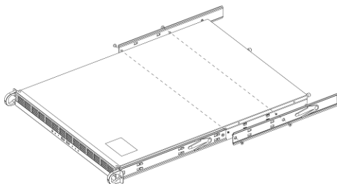
① Fixer les rails intérieurs et du serveur
