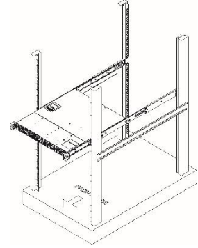
③ Встановіть сервер у стійку
