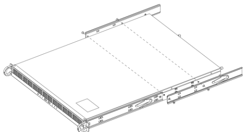
① Fissare il server e i binari interni
