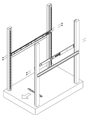
② Installeer de buitenrails
