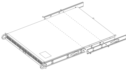
① Pasang Server dan Rel Dalam
