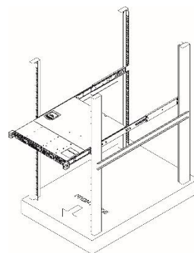
③ Helyezze a szervert az állványra
